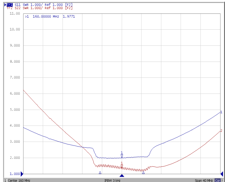
VSWR
